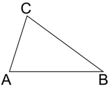
Triangolo acutangolo scaleno
