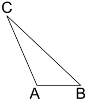
Triangolo ottusangolo scaleno
