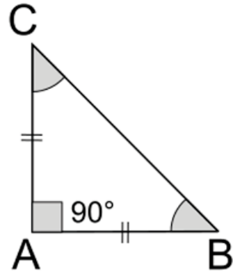
Triangolo rettangolo isoscele
