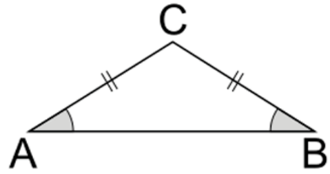
Triangolo ottusangolo isoscele
