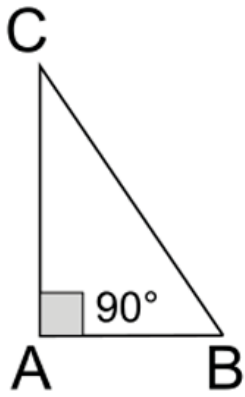
Triangolo rettangolo scaleno
