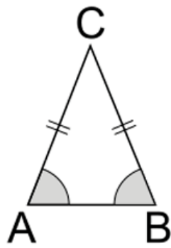
Triangolo acutangolo isoscele
